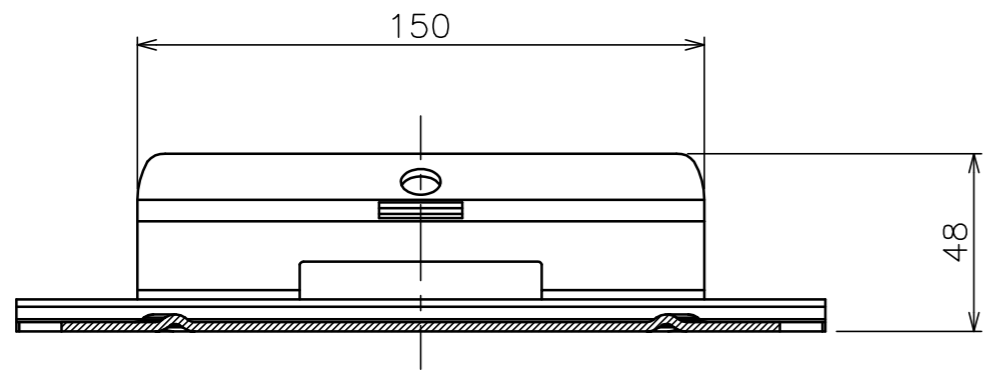
B-B 断面
