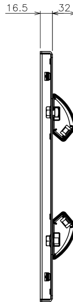
A-A 断面
