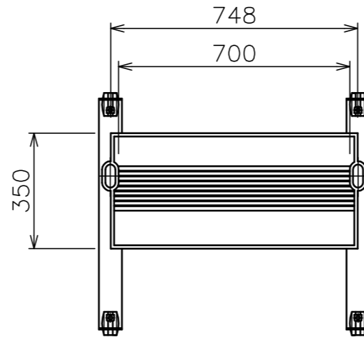
X-X矢視図
