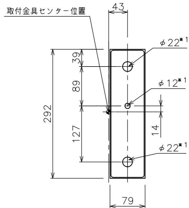
壁面取り付け穴-3寸法図
