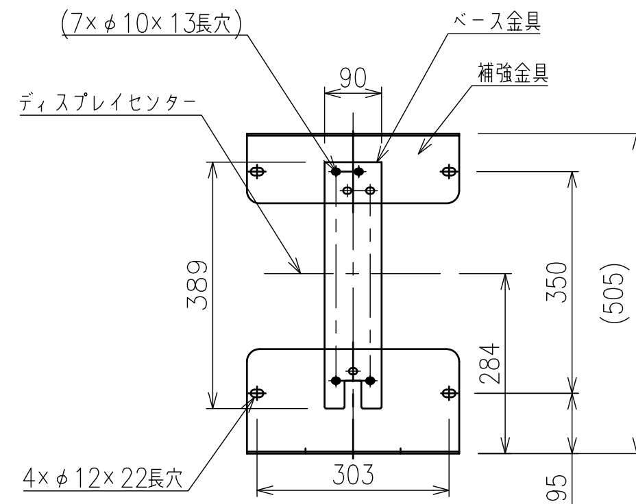
ベース金具正面図
