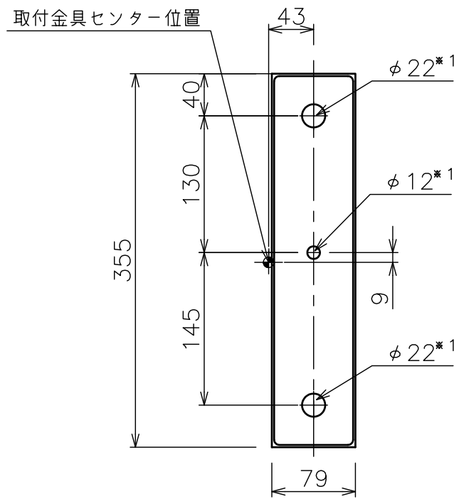
壁面取り付け穴寸法図
