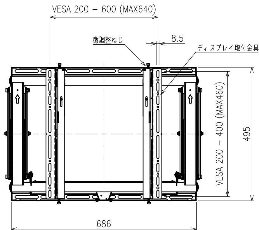
ディスプレイ取付穴位置 拡大図
