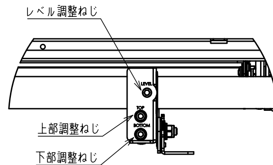
A部分詳細図 S=1/4
