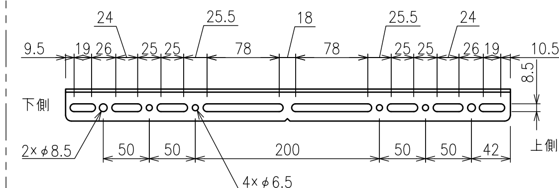
ディスプレイ取付穴位置 拡大図
