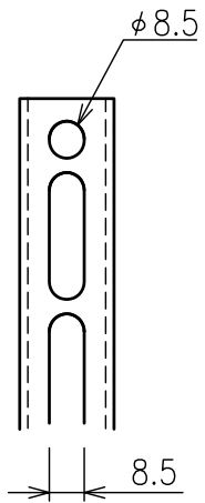
A部分拡大図 S=1/2
